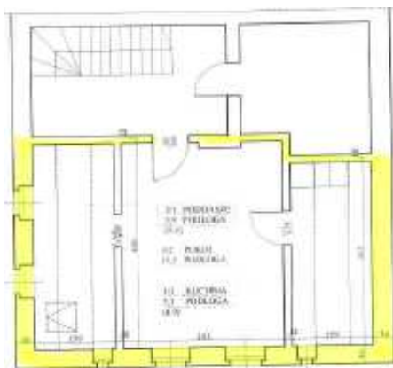
Rzut poddasza
